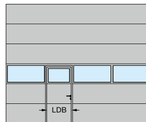
SPU F42 / SPU 67 Thermo Cadres en Alu Portillon incorporé disposé à gauche
