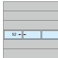
SPU F42 / SPU 67 Thermo Cadres en Alu Répartition homogène des compartiments
