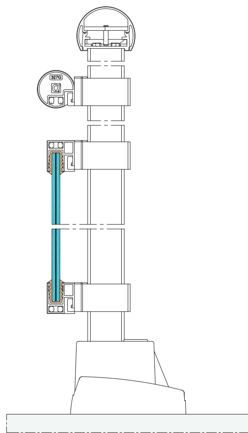
Coupe verticale
