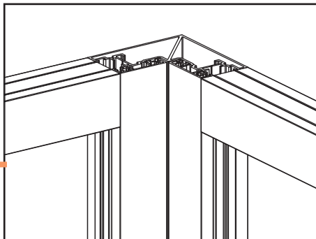
Assemblage cadre et poteau 2 départs Frame and 2D post assembly
